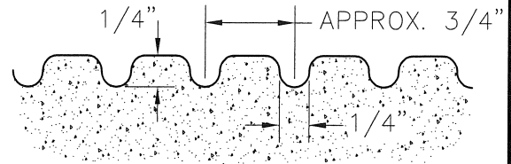
TACTILE GROOVE DETAIL N.T.S.
